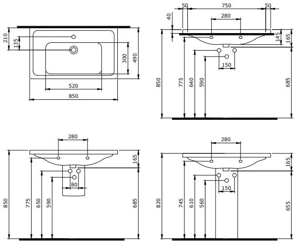
1008-001-0126 Taormina Pro Etajerli Lavabo 85 cm Taormina Pro Washbasin 85 cm Taormina Pro Lavabo 85 cm
