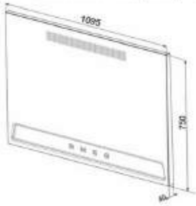
KITCFE120X (CFE120 serisi portafino kuzineler için ortak çizim)
